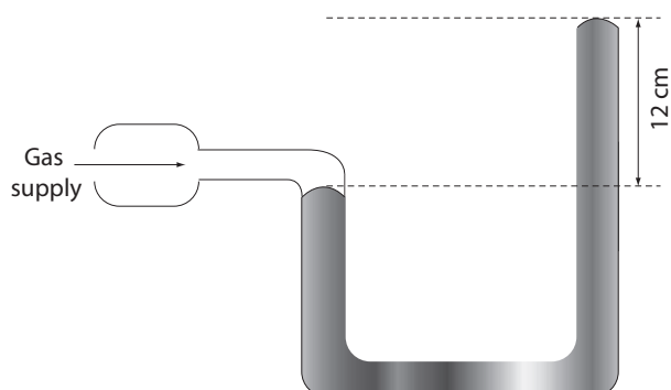
Fig. 8.11 : U-tube manometre
