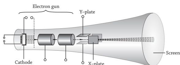
Fig 22.8 : Cathode ray oscilloscope
