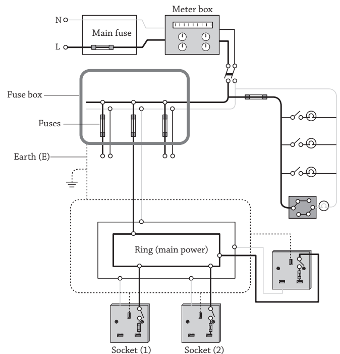
Fig 18.23 : House wiring
