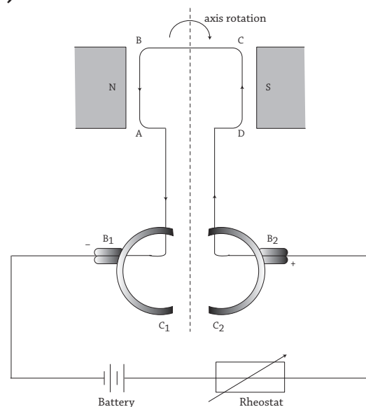
Fig 20.11 : A d.c. motor
