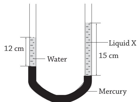
Fig 8.4 : U-tube manometer
