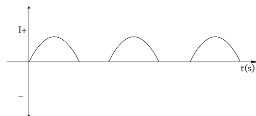
Fig 21.8 (b) : Half-wave rectification
