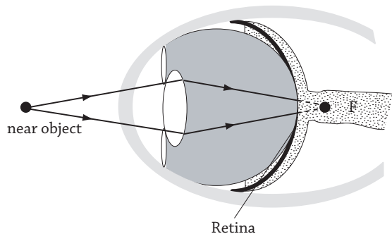
Fig 12.41 : Long-sightedness
