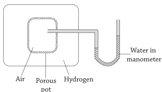
Fig 4.6 : Diffusion of gases
