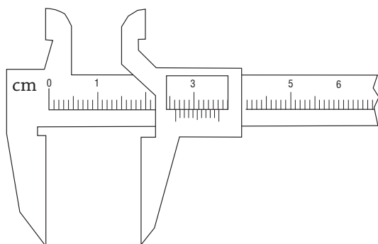
Fig. 6.4 (a) : A vernier callipers
