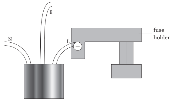
Fig 18.22 : A plug
