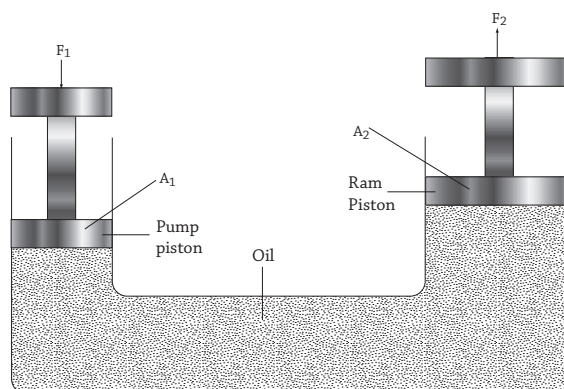
Fig 8.6 : Hydraulic press
