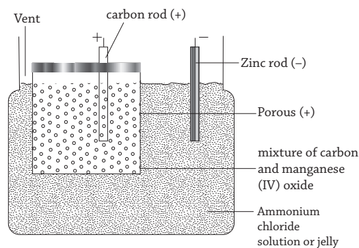
Fig 17.8 : A wet leclanche cell
